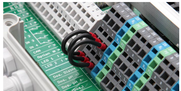
Pontages à fil dans le bornier de la phase L D au contact central de relais a
